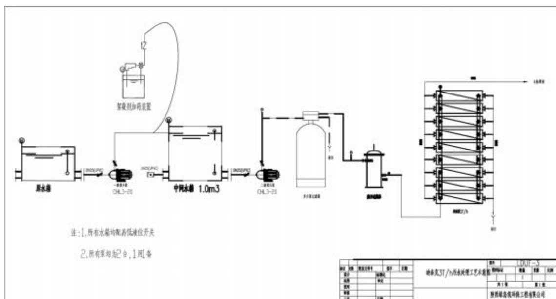
图 4-1 废水处理设施（絮凝沉降+多介质过滤+微孔折叠过滤+超滤）图
