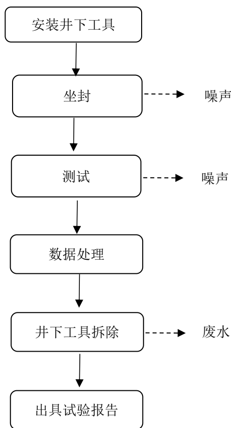
图 2-2 封隔器和桥塞气密封测试平台试验流程及产污环节图
