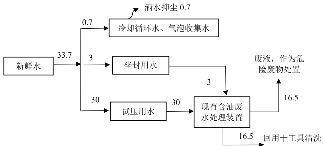
图 2-1 项目运营期水平衡图 (单位: \text{m}^3/\text{a} )
