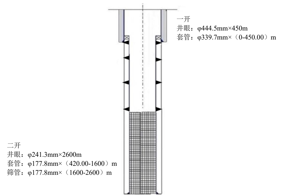
图 2-6 回灌井（直井）井身结构示意图
