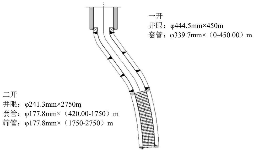
图 2-5 生产井（定向井）井身结构设计示意图
