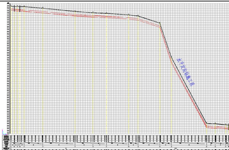
图 2.4 水平定向钻施工
