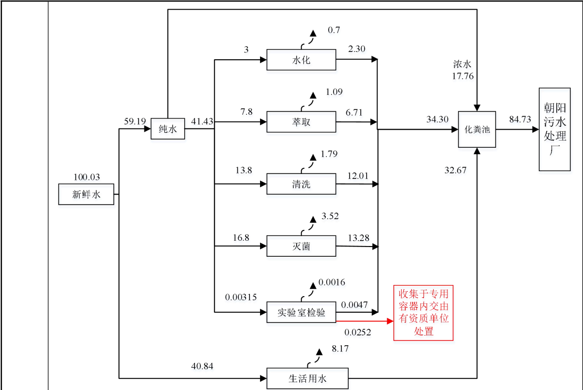
图 2-2 扩建后全厂水平衡图 单位：m³/d
