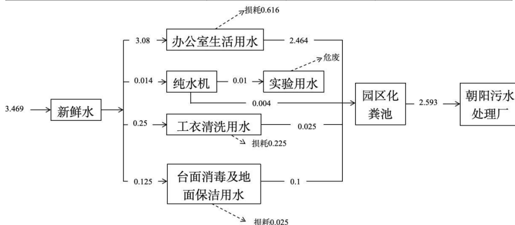
图 4 项目水平衡图 单位: \text{m}^3/\text{d}
