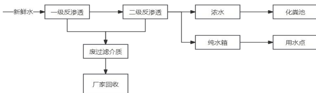
图 6 超纯水制备工艺流程及产污环节图
