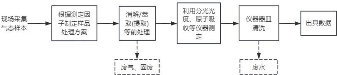
图 2-4 气态样品实验流程及产污环节图
