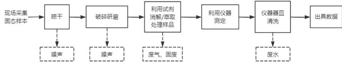
图 5 固态样品实验流程及产污环节图
