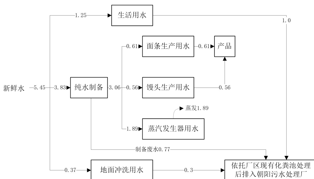
图 2-1 项目水平衡图 单位: \text{m}^3/\text{d}
