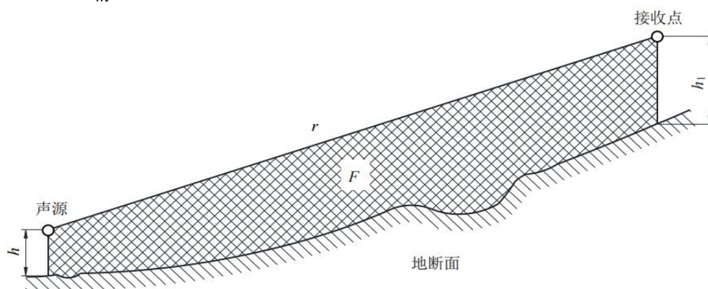
图 5.2 估计平均高度 h_m 的方法 ( h_m = F/r )
