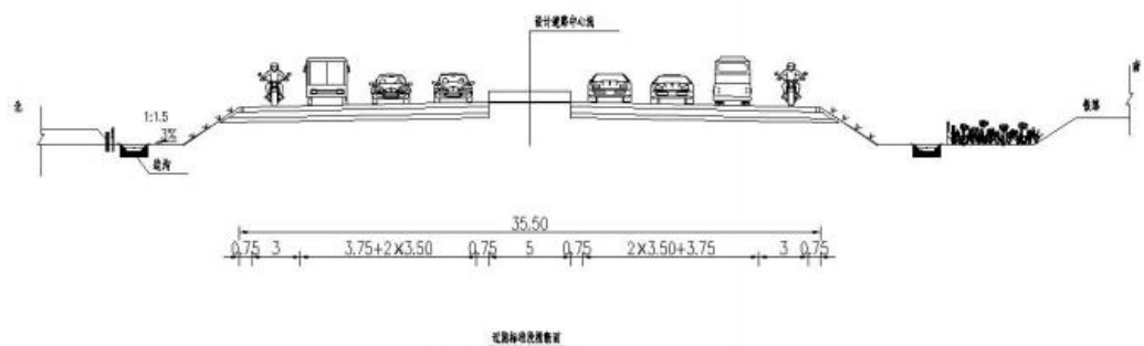
图 2-1 近期标准段横断面
