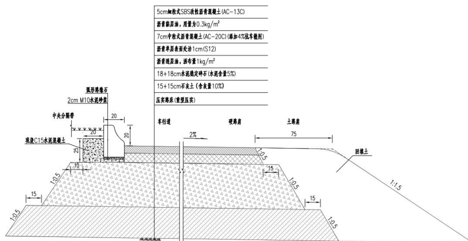
图 2-3 车行道及硬路肩路面结构示意图
