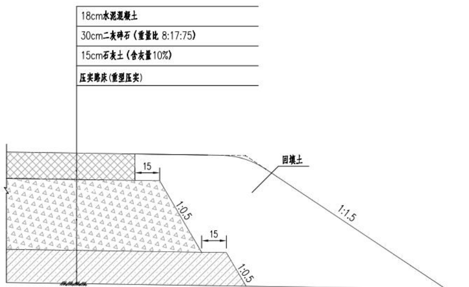
图 2-4 村道路面结构示意图
