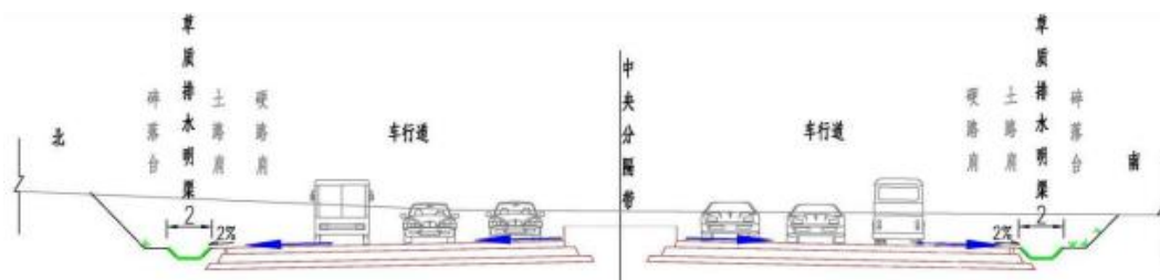
图 2-5 道路横向排水示意图
