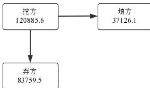
图 2-9 土石方平衡图（单位：m 3 ）
