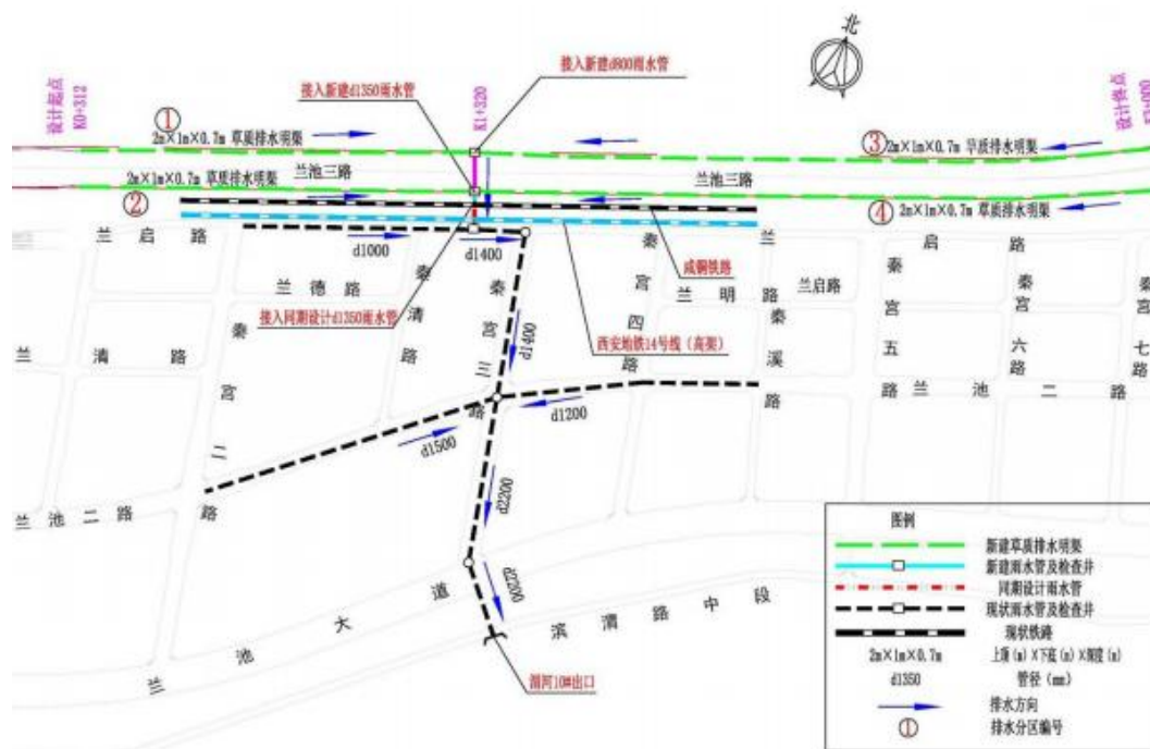
图 2-6 排水分区示意图
