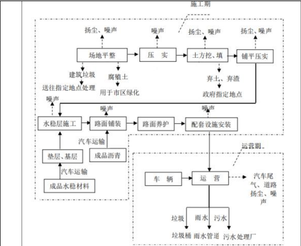
图 2-11 施工工艺流程图
