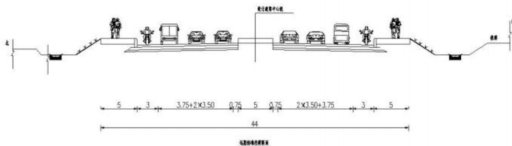
图 2-2 远期标准段横断面
