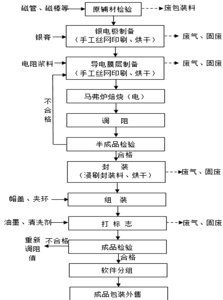
图5 玻璃釉电阻器生产工艺及产污环节图
