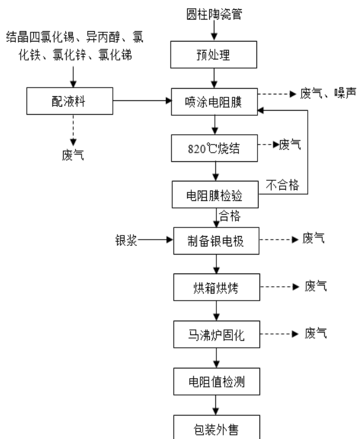
图4 氧化膜电阻器生产工艺及产污环节图
