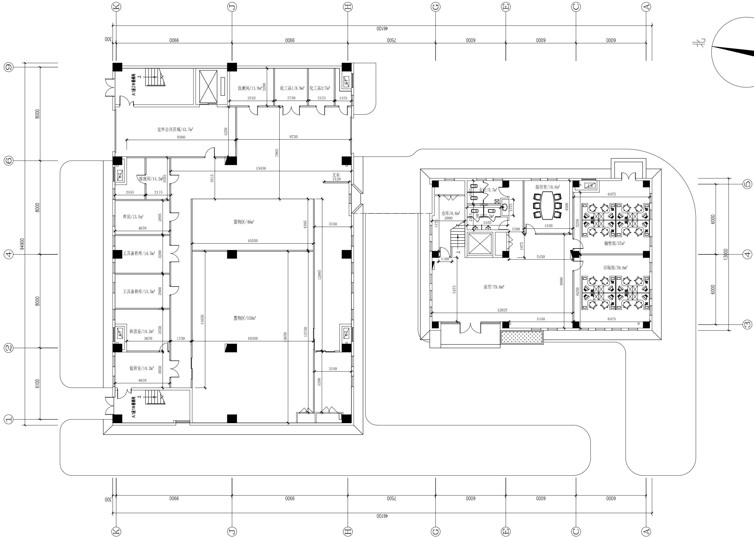
一层平面布置图
