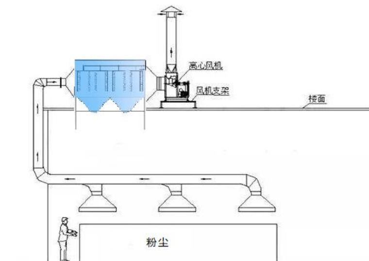
图4-1 粉尘产生、收集和治理、排放示意图
