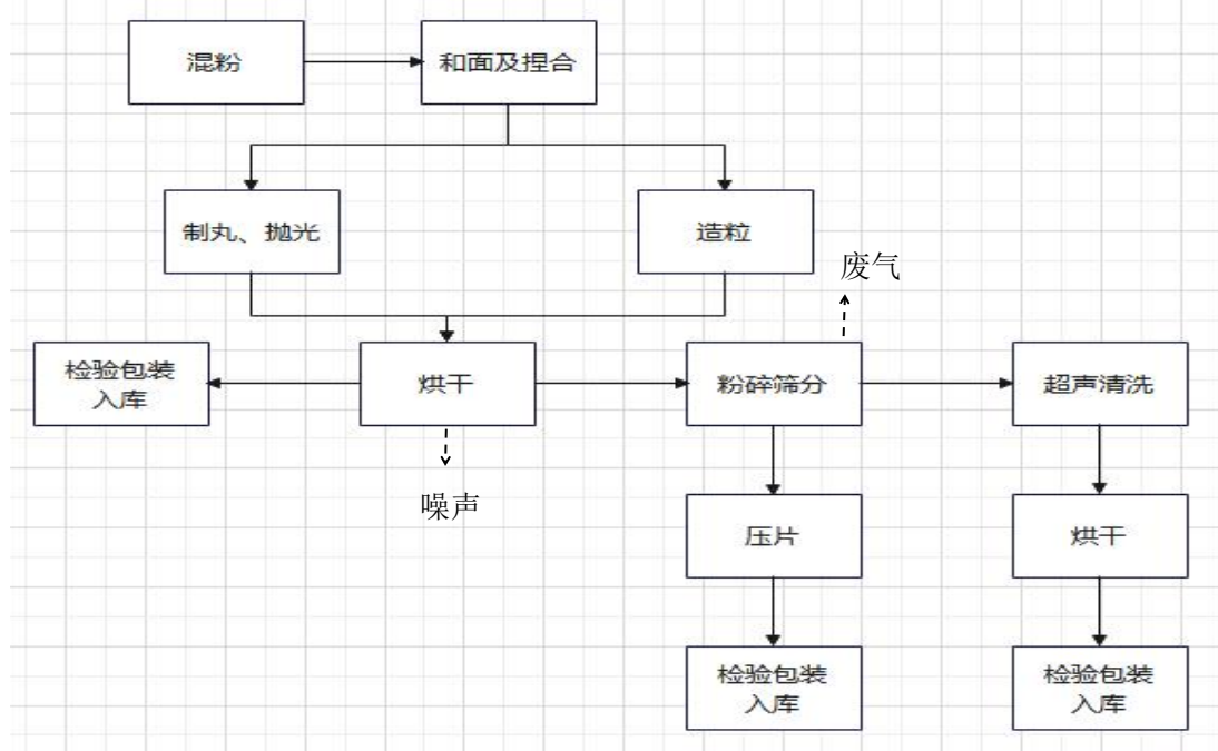
图 2-5 活性炭阻垢材料及抑菌阻垢材料工艺流程
