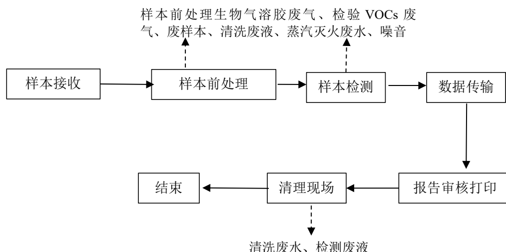
图 10 质谱检测工艺流程图
