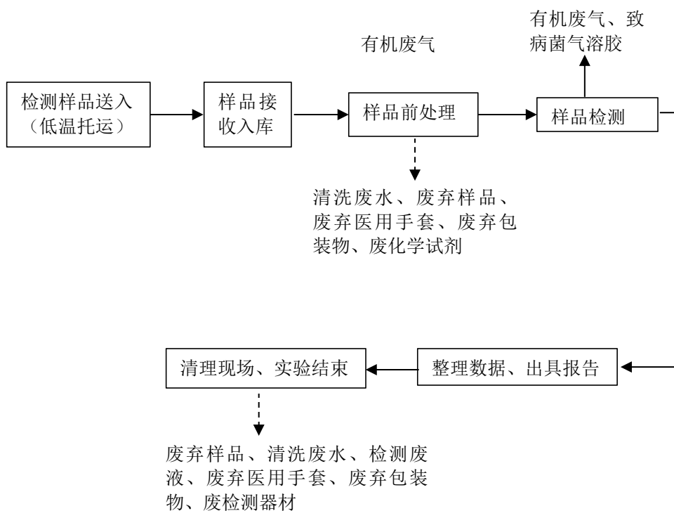
图 2 项目整体检验过程工艺流程图
