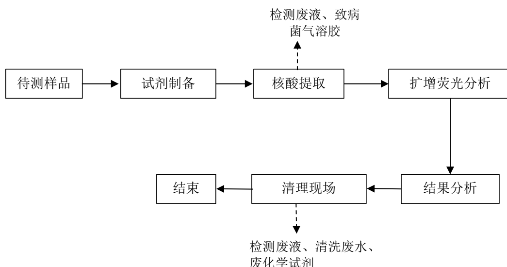
图 6 PCR 检测过程工艺流程图
