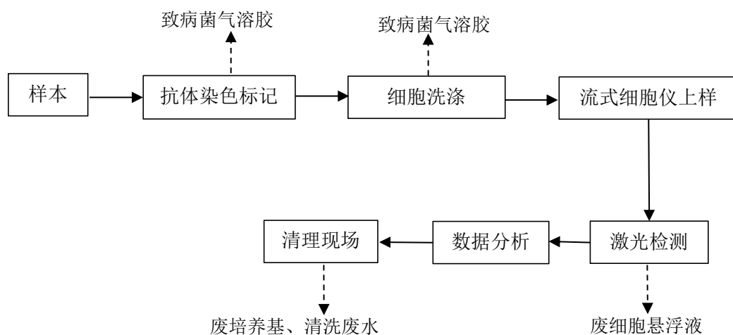
图 5 流式细胞实验工艺流程图
