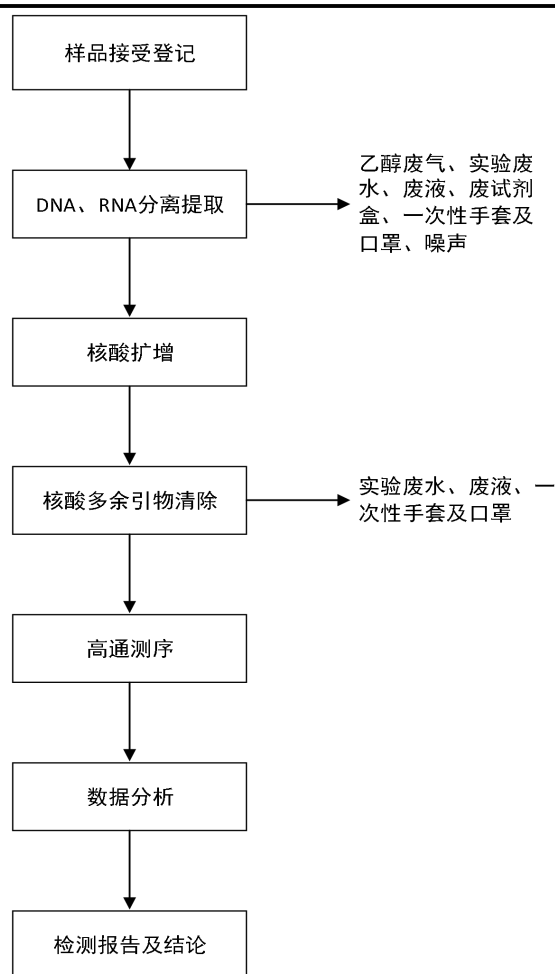
图 11 NGS 程技术中心-基因检测工艺流程图
