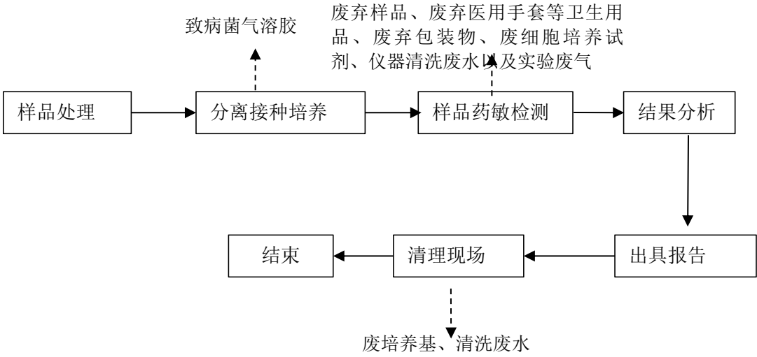
图 13 器官工程技术中心工艺流程图
