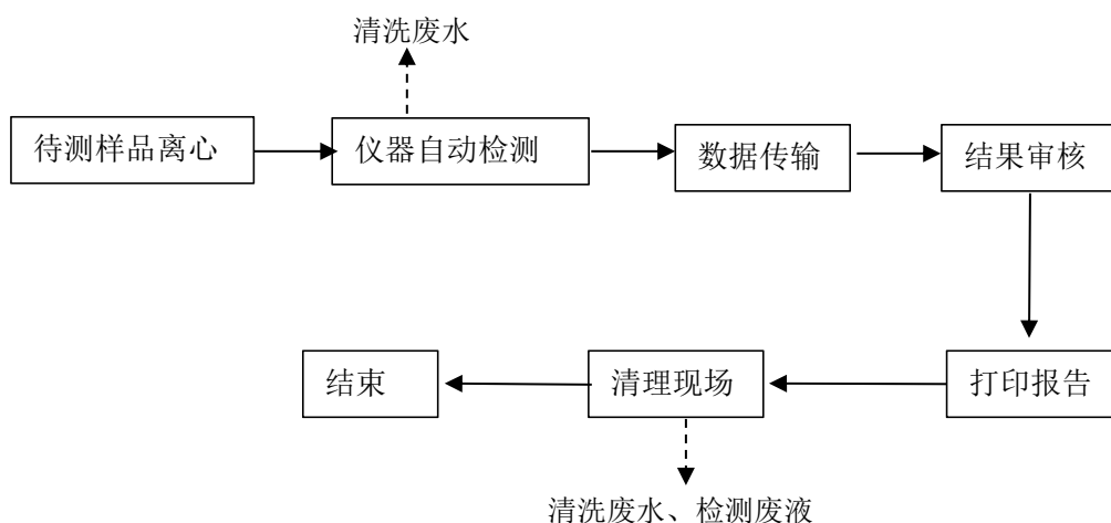
图 8 仪免、生化检测过程工艺流程图
