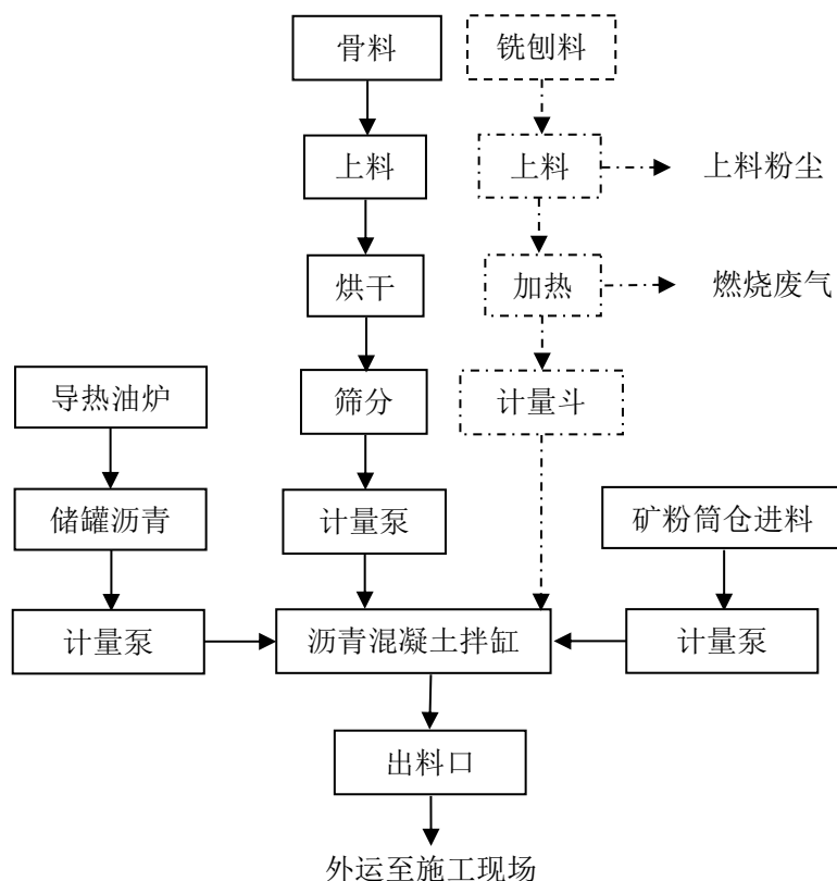
图 2-1 运营期生产工艺流程及产污环节图
