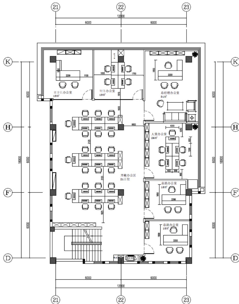
附图 3-3 办公楼三层平面布置图
