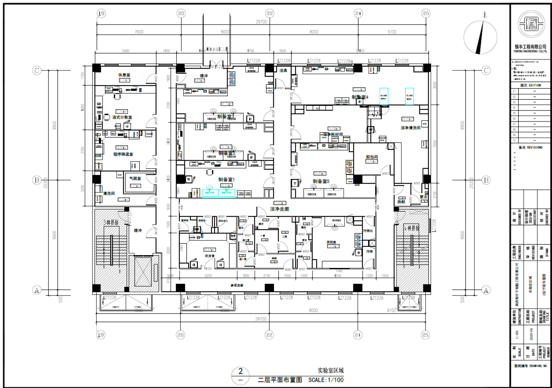
附图 2-2 实验楼二层平面布置图
