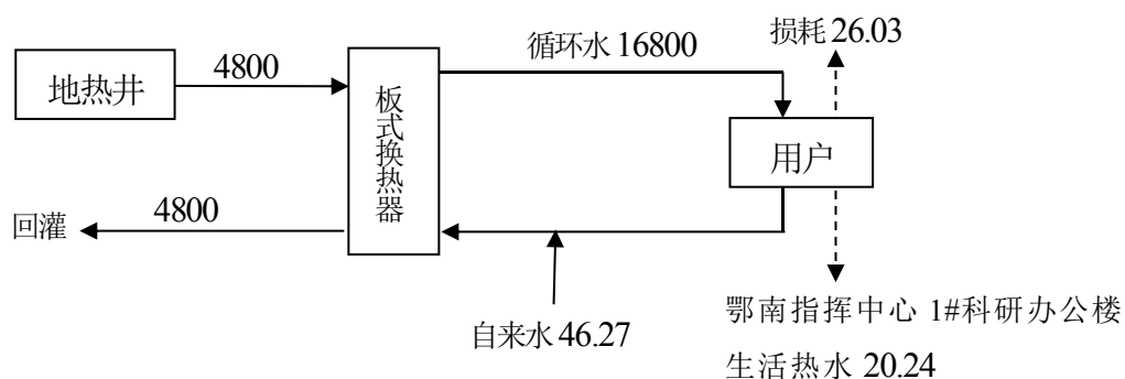
图 5 项目生产用水水量平衡图
