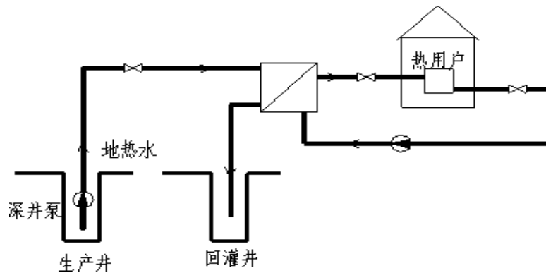
图 1 地热间接式供热系统示意图
