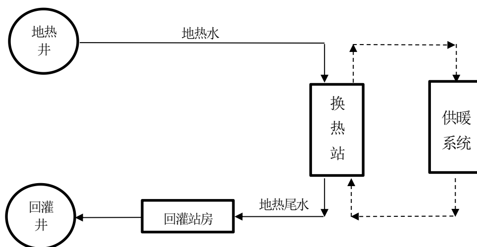
图3 项目运营期工艺流程图
