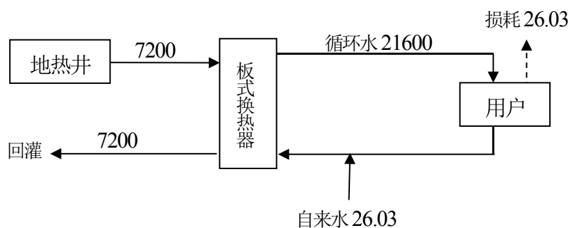
图 5 项目生产用水水量平衡图
