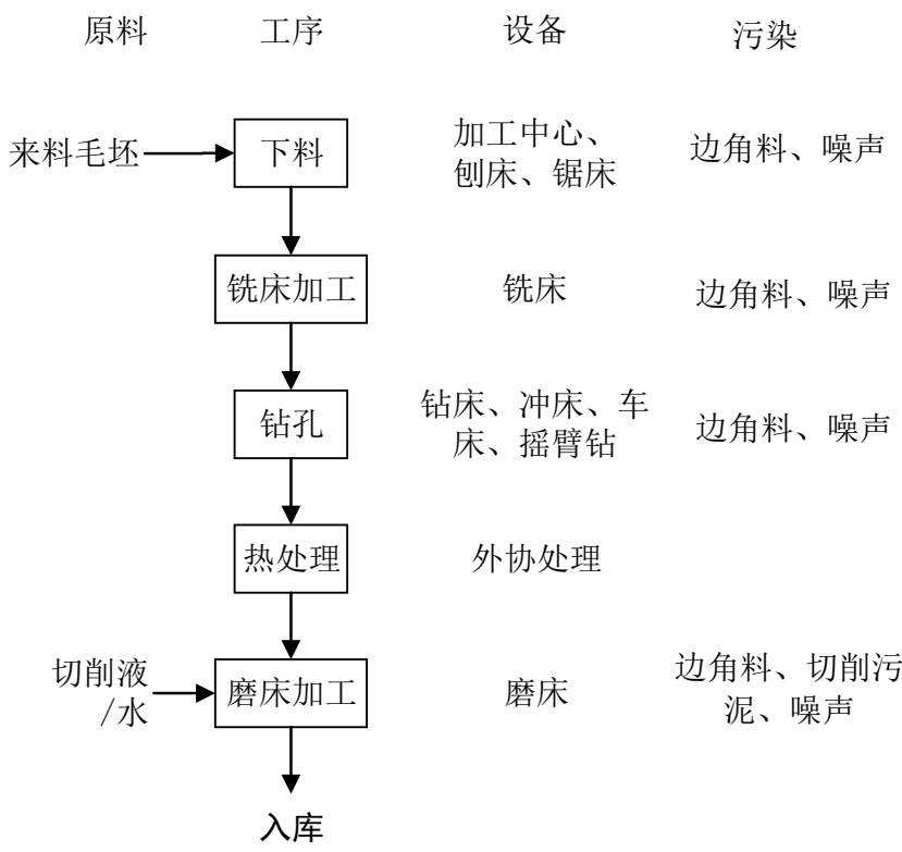
图 3 项目生产工艺流程及产污环节图
