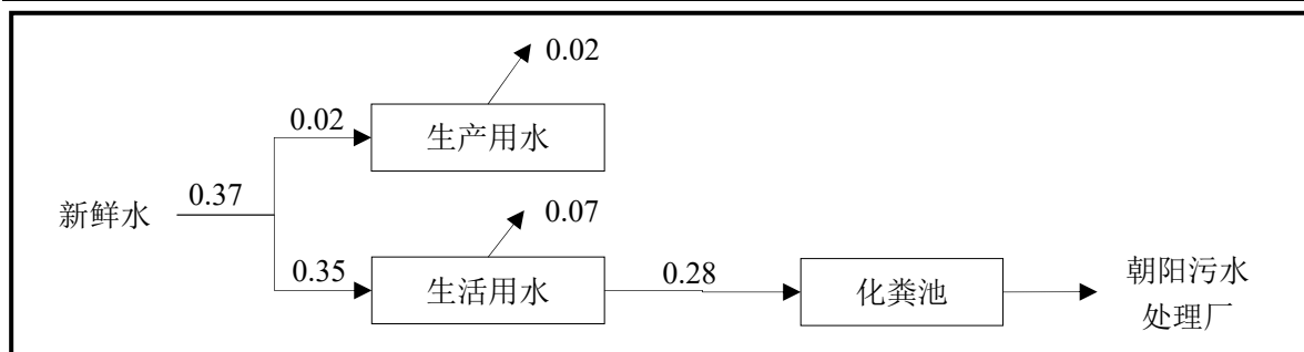
图 1 项目水平衡图 单位： \text{m}^3/\text{d}
