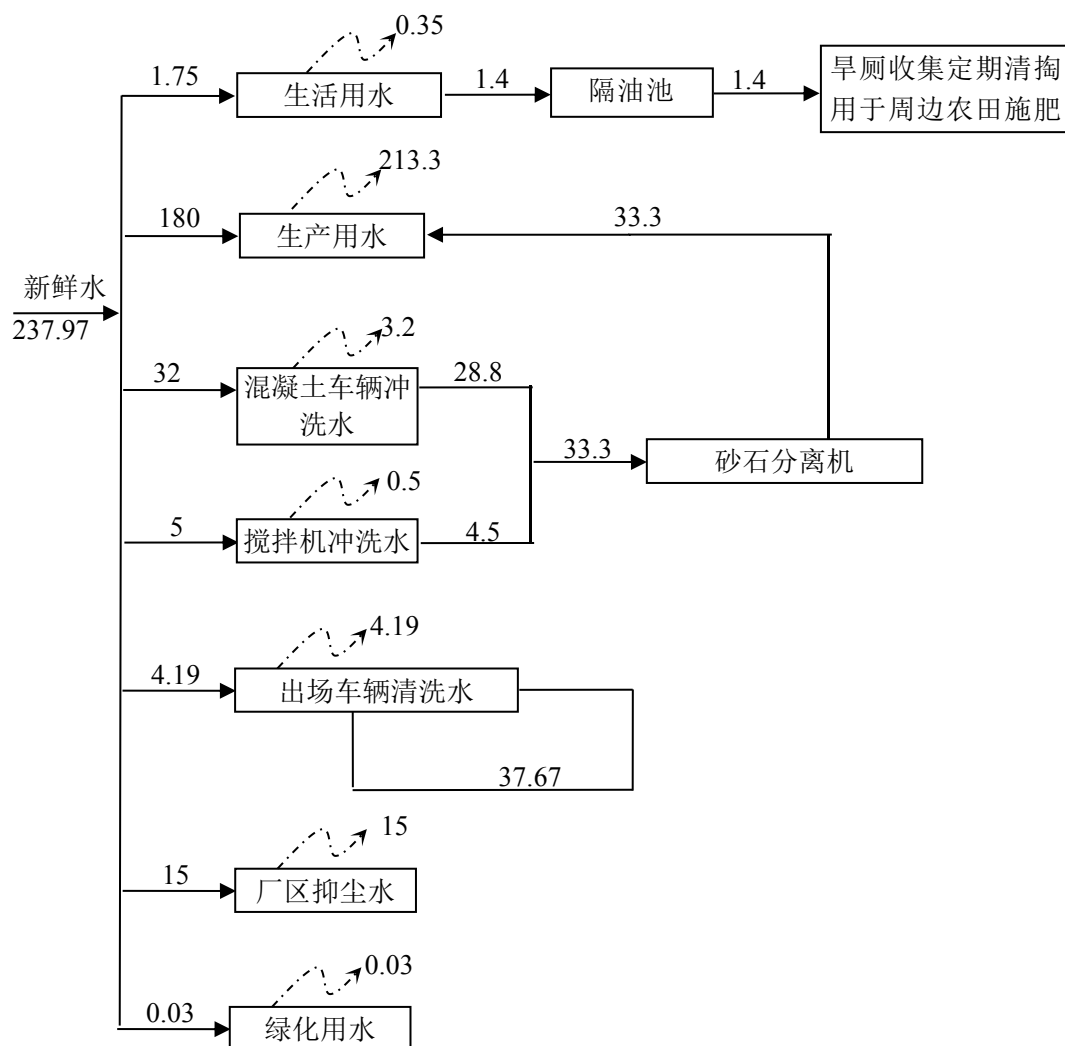
图 2 项目水平衡图 (m³/d)
