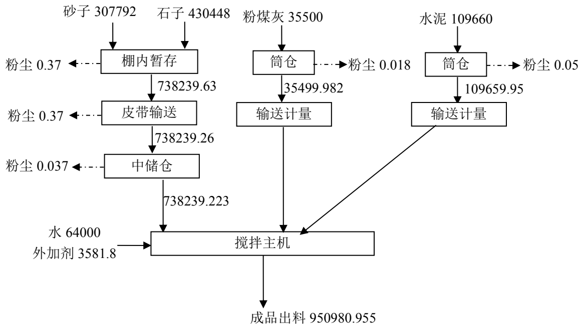
图 1 物料平衡图 t/a
