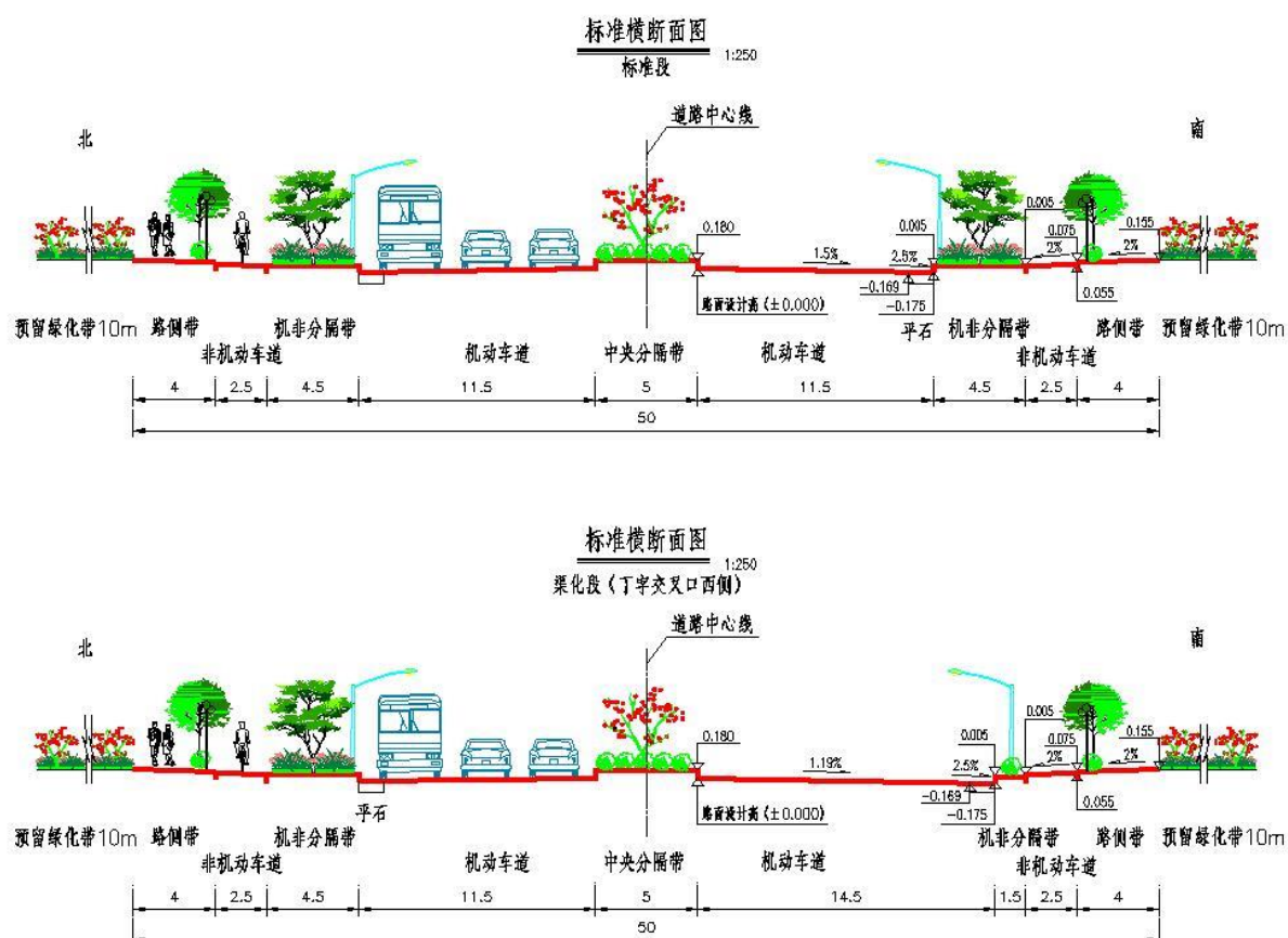
图 1 道路横断面示意图
