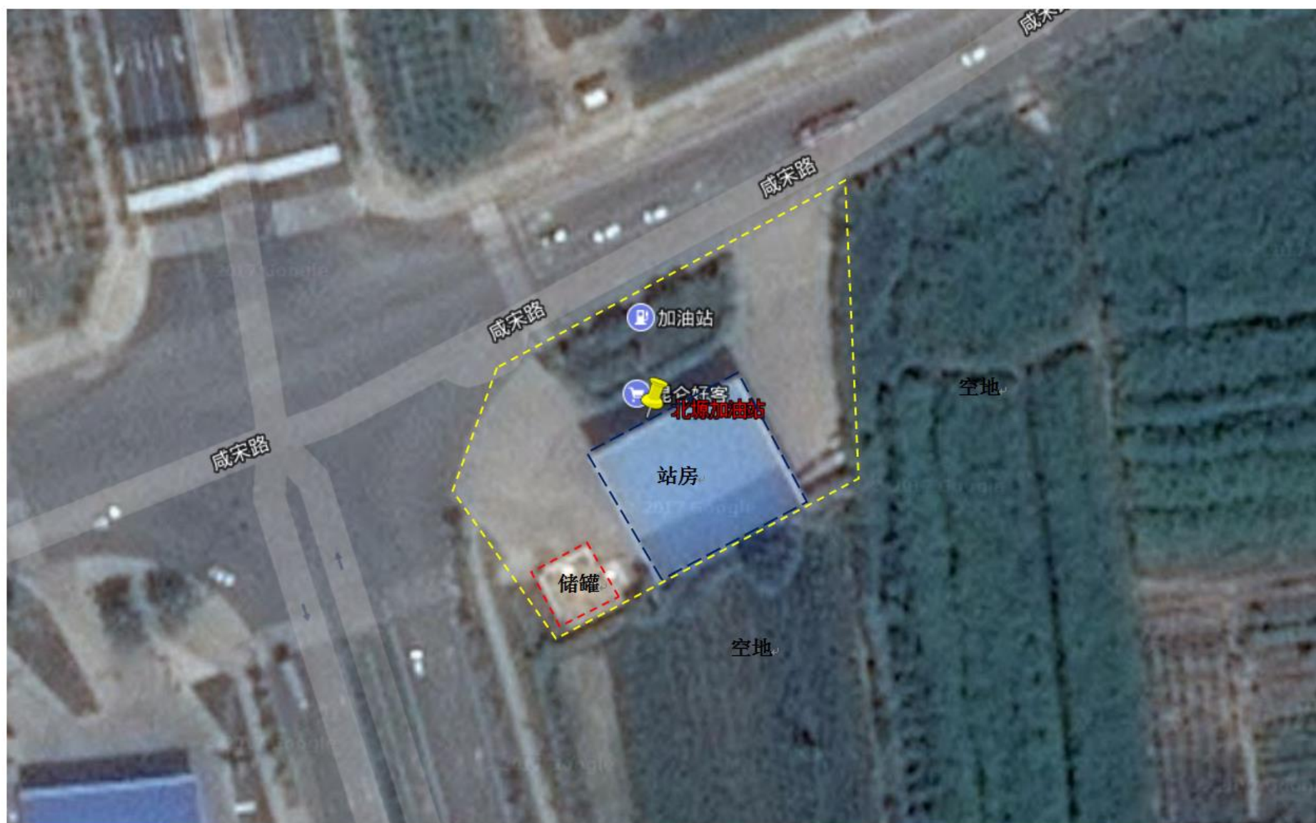
附图 2 加油站平面布置及四邻关系图
